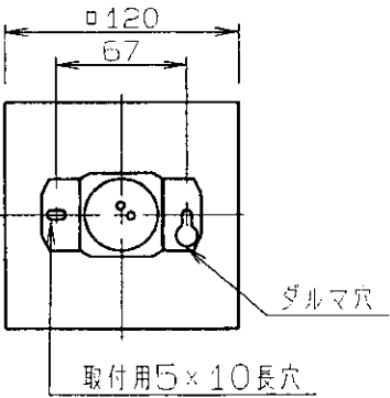
取付寸法(矢視a)
