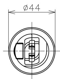
取付寸法（矢視 ②）
