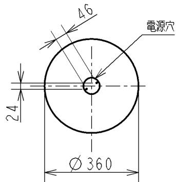
取付寸法 ( 矢視 ④ )
