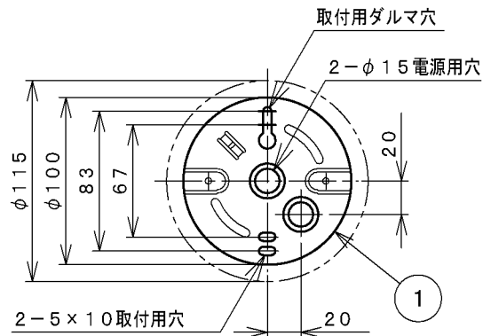
取付寸法（矢視a）
