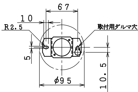
取付寸法(矢視 ㊸)
