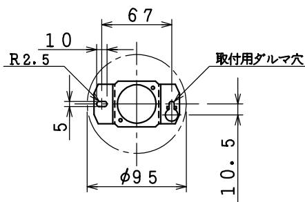
取付寸法(矢視 ㊟)
