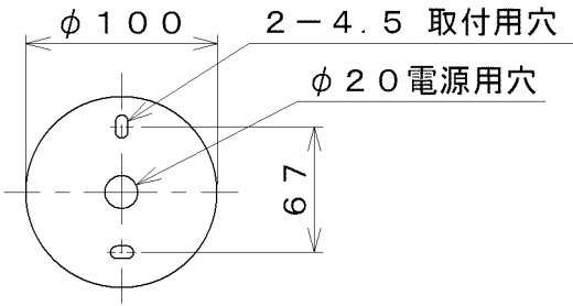
取付寸法(矢視①)
