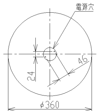
取付寸法（矢視 ①）
