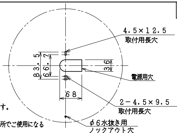
取付寸法(矢視 ⑥)
