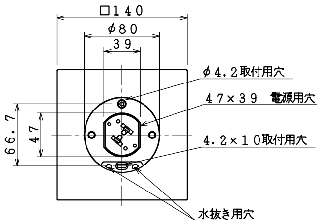
取付寸法(矢視 ②)
