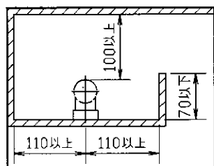
<施工最小寸法・床付>
