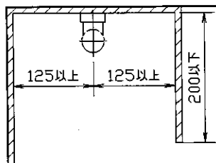
<施工最小寸法・直付>
