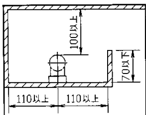
<施工最小寸法・床付>
