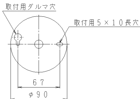
取付寸法（矢視②）
