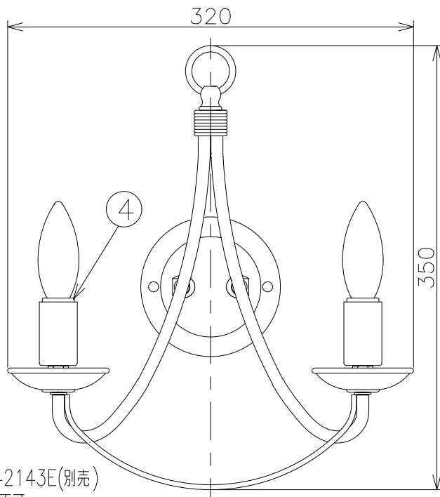
取付寸法 (矢視 (a))
