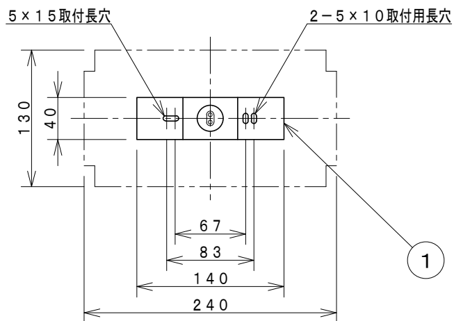
取付寸法 (矢視 a)
