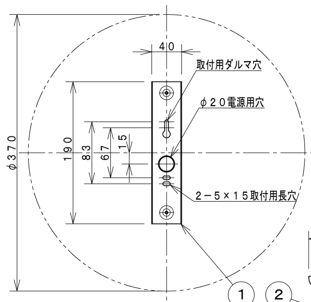
取付寸法 (矢視 a)
