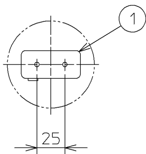
取付寸法 矢視 ㊤
