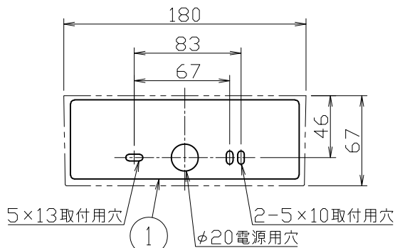
取付寸法（矢視 ①）
