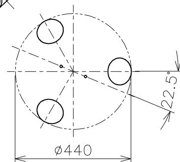
灯具配置/取付角度 (下面ヨリ)
