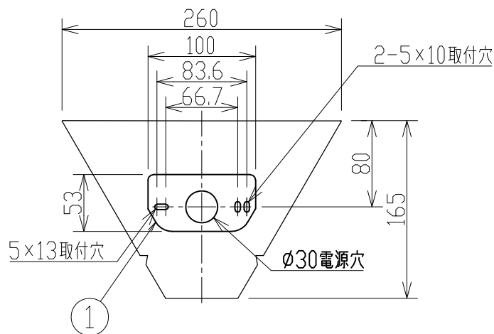
取付寸法(矢視a) (縮尺1/5)
