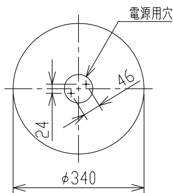
取付寸法(矢視 ㊟)
