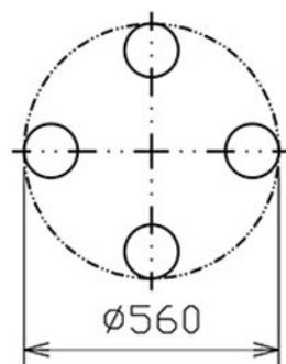
灯具配置図
