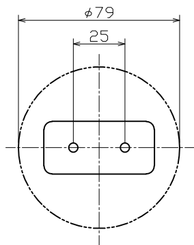
取付寸法（矢視④）
