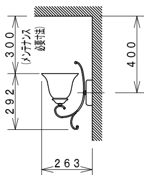
取付寸法 (矢視 a)
