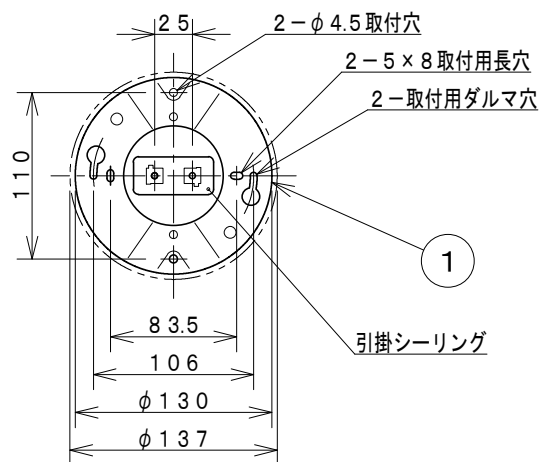
取付寸法 (矢視 a)
