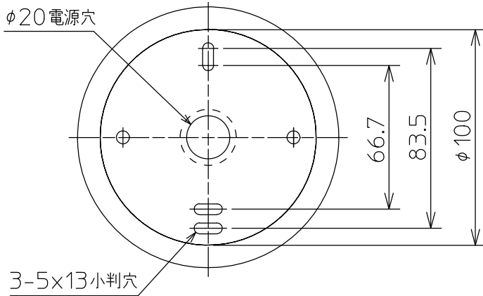
取付寸法（矢視a）
