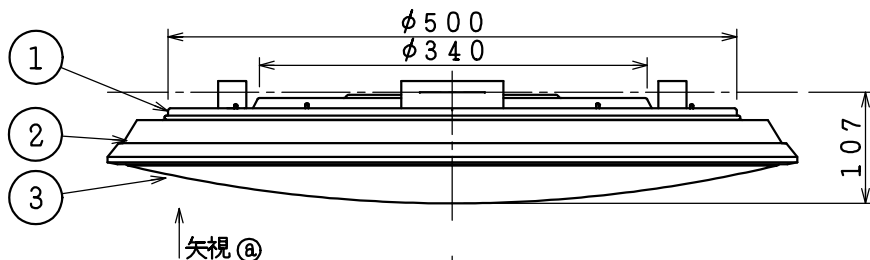
取付寸法(矢視 a)
