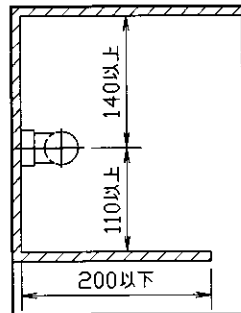
<施工最小寸法・壁付>
