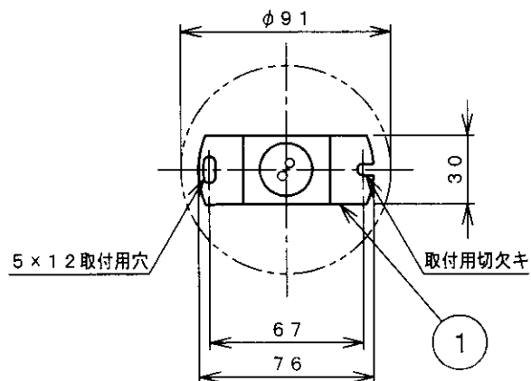
取付寸法（矢視a）
