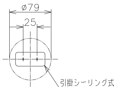
取付寸法 (矢視 ㊸)
