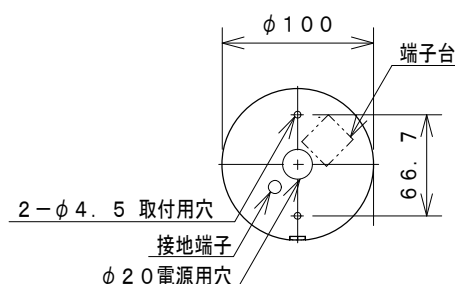
取付寸法(矢視a)
