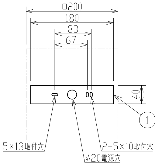
取付寸法(矢視a) (縮尺1/5)
