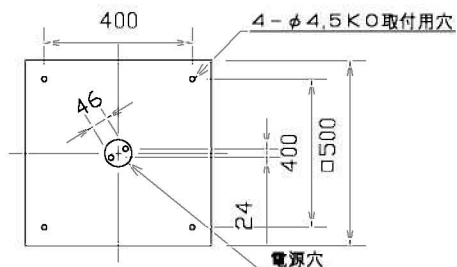
取付寸法〔矢視 (a)〕
