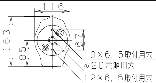
取付寸法 (矢視 ①)
