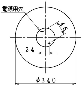
取付寸法 (矢視 ①)
