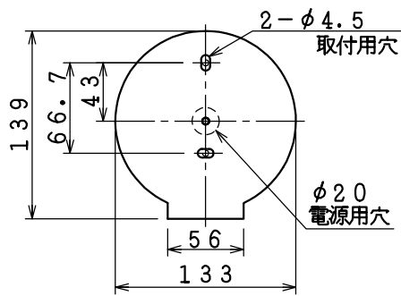
取付寸法 ( 矢視 ④ )
