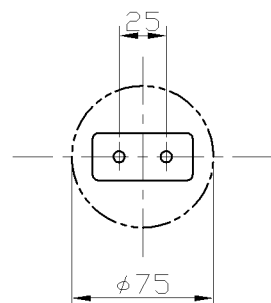
取付寸法（矢視α）
