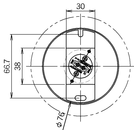
取付寸法（矢視②）
