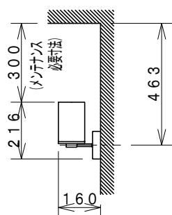
取付寸法 (矢視 a)
