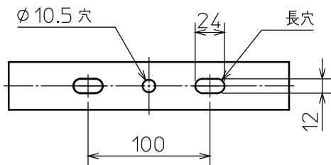
取付寸法(矢視 ㊤)
