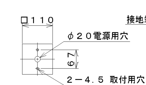
取付寸法(矢視@)
