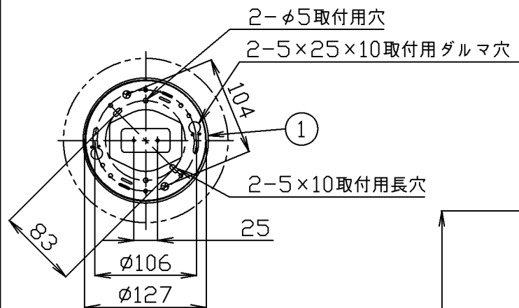
取付寸法 (㊤ 矢視)
