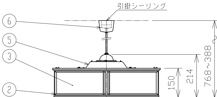
取付寸法（矢視 ①）
