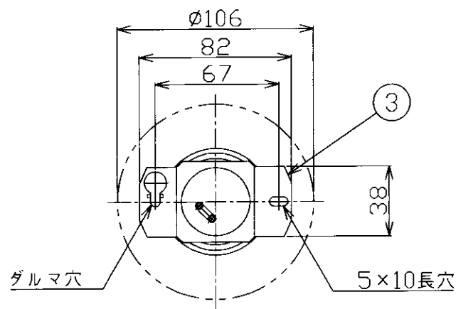
取付寸法 (矢視 ㊤)
