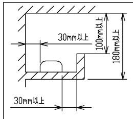
最小施工寸法
