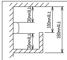
最小施工寸法
