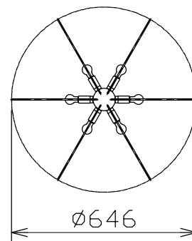
灯具配置図
