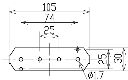
取付寸法(矢視 a) (縮尺1/3)
