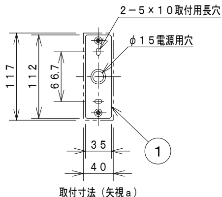
取付寸法 (矢視 a)
