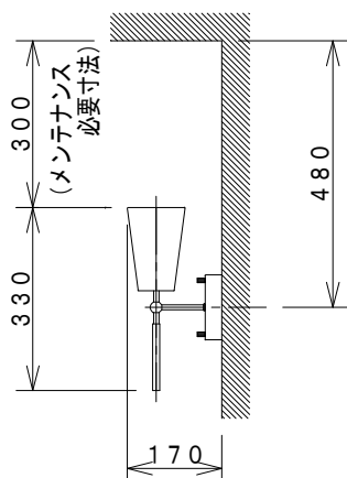
取付寸法 (矢視 a)
