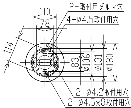
取付寸法(矢視 ㊟)
