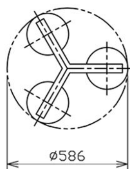
灯具配置図
